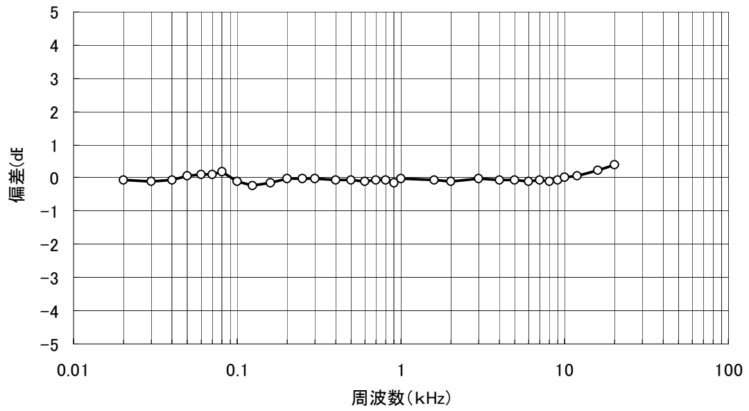
RIAA偏差特性
