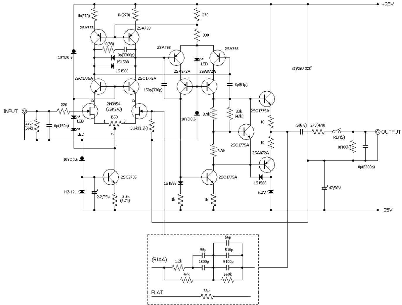
アンプ部回路図
