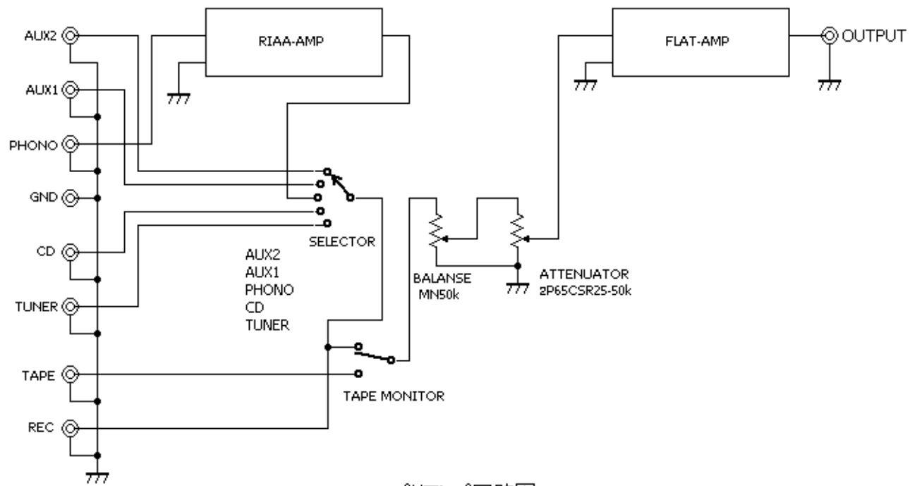
プリアンプ回路図
