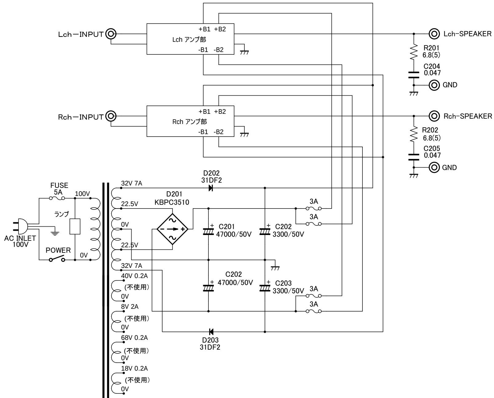
全体回路
