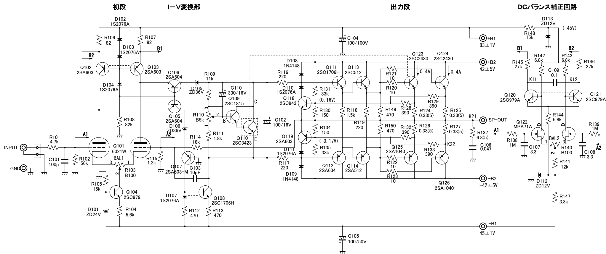
AMP-1509A パワーアンプ回路例
