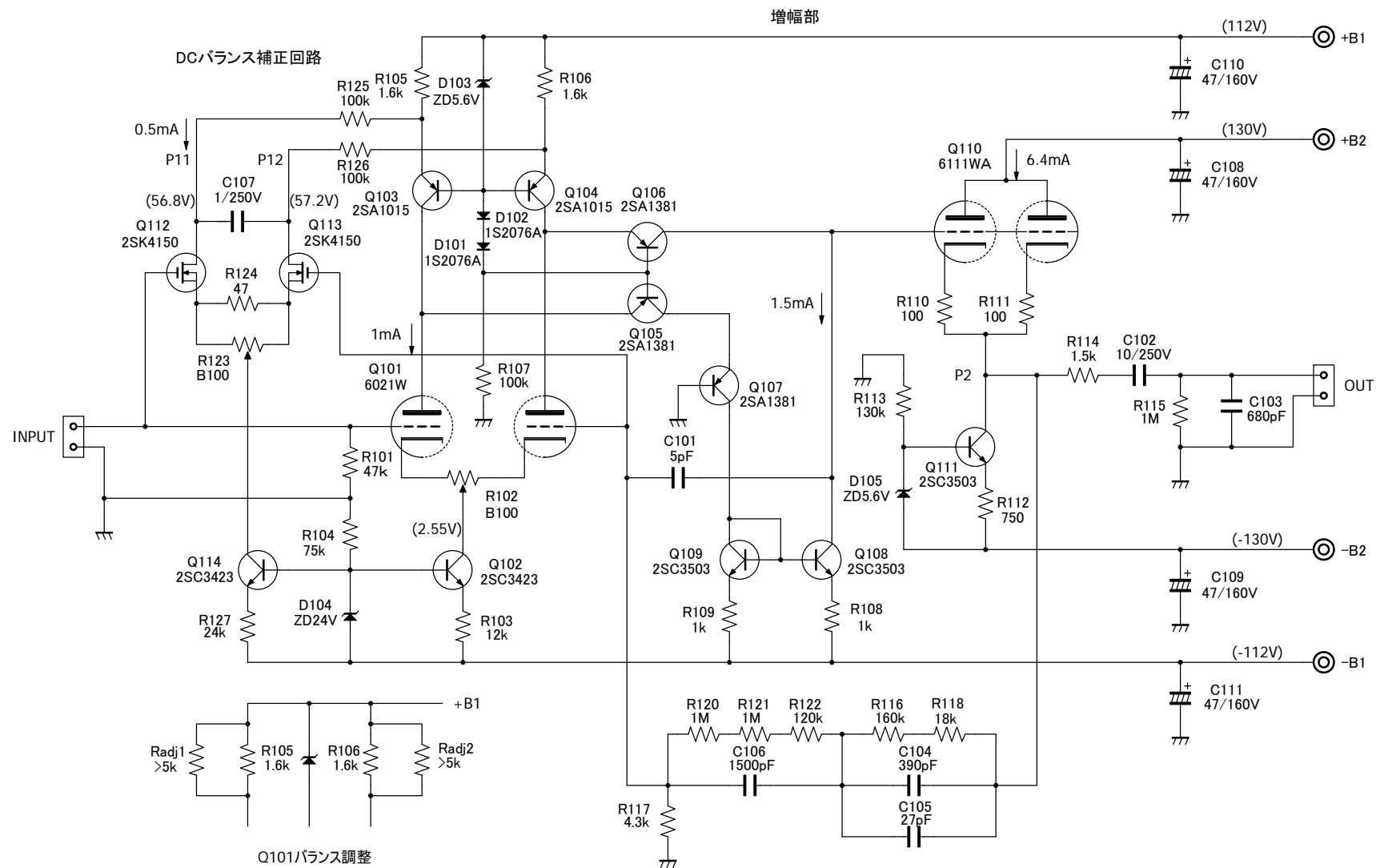
EQ-1505A イコライザーアンプ回路例
