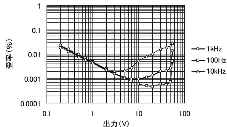
フラットアンプ歪率特性(ゲイン20dB)
