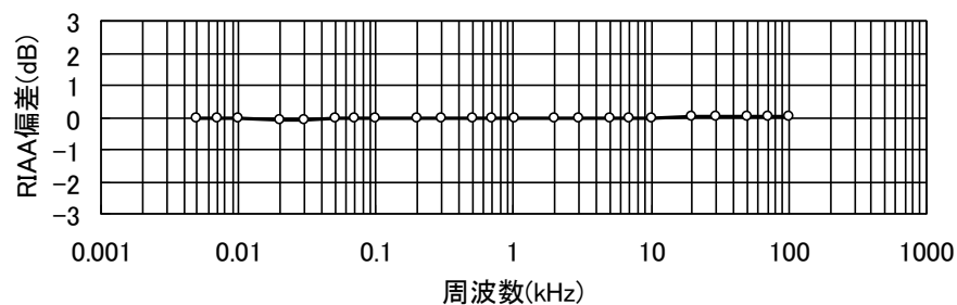
RIAA偏差
