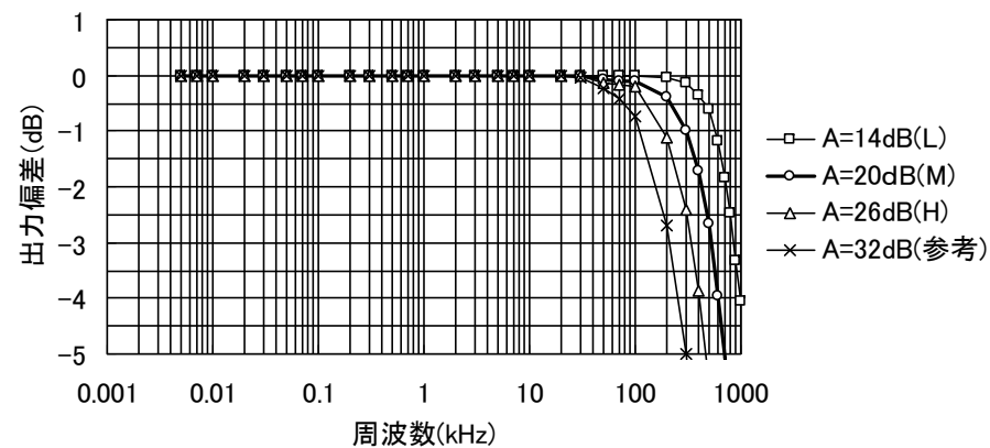
フラットアンプ周波数特性
