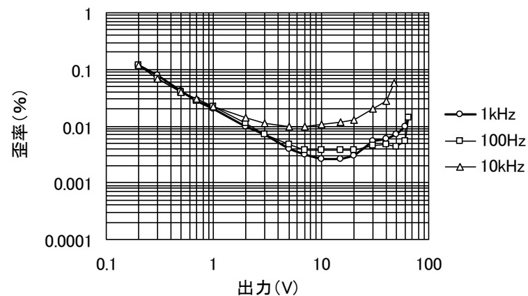
イコライザーアンプ歪率特性
