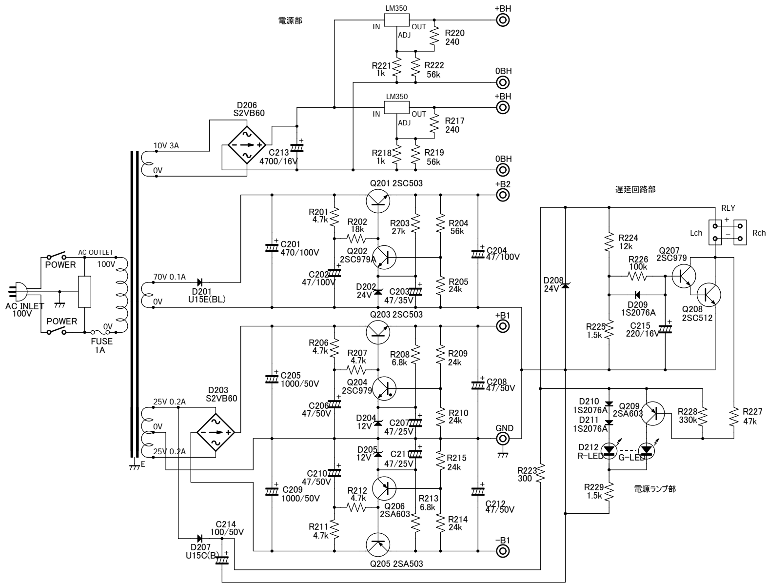
PS-1401B 電源回路例
